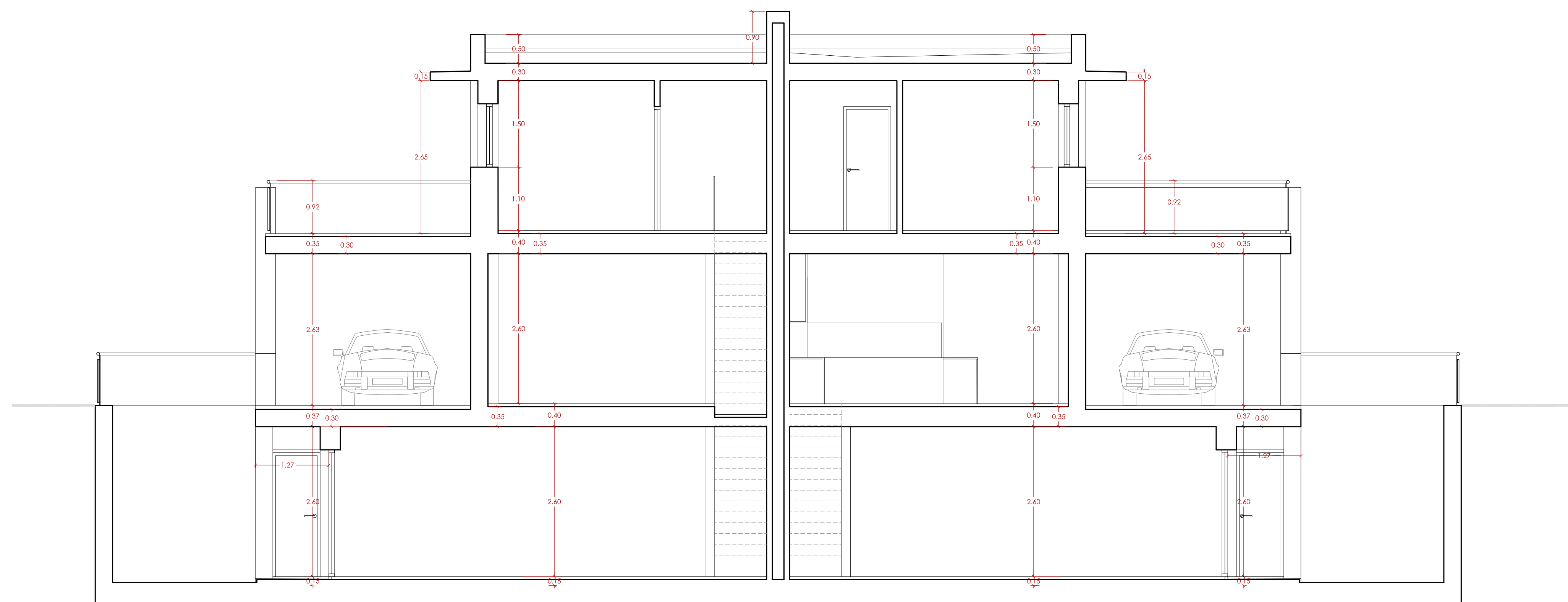
SECCIÓN B-B'
