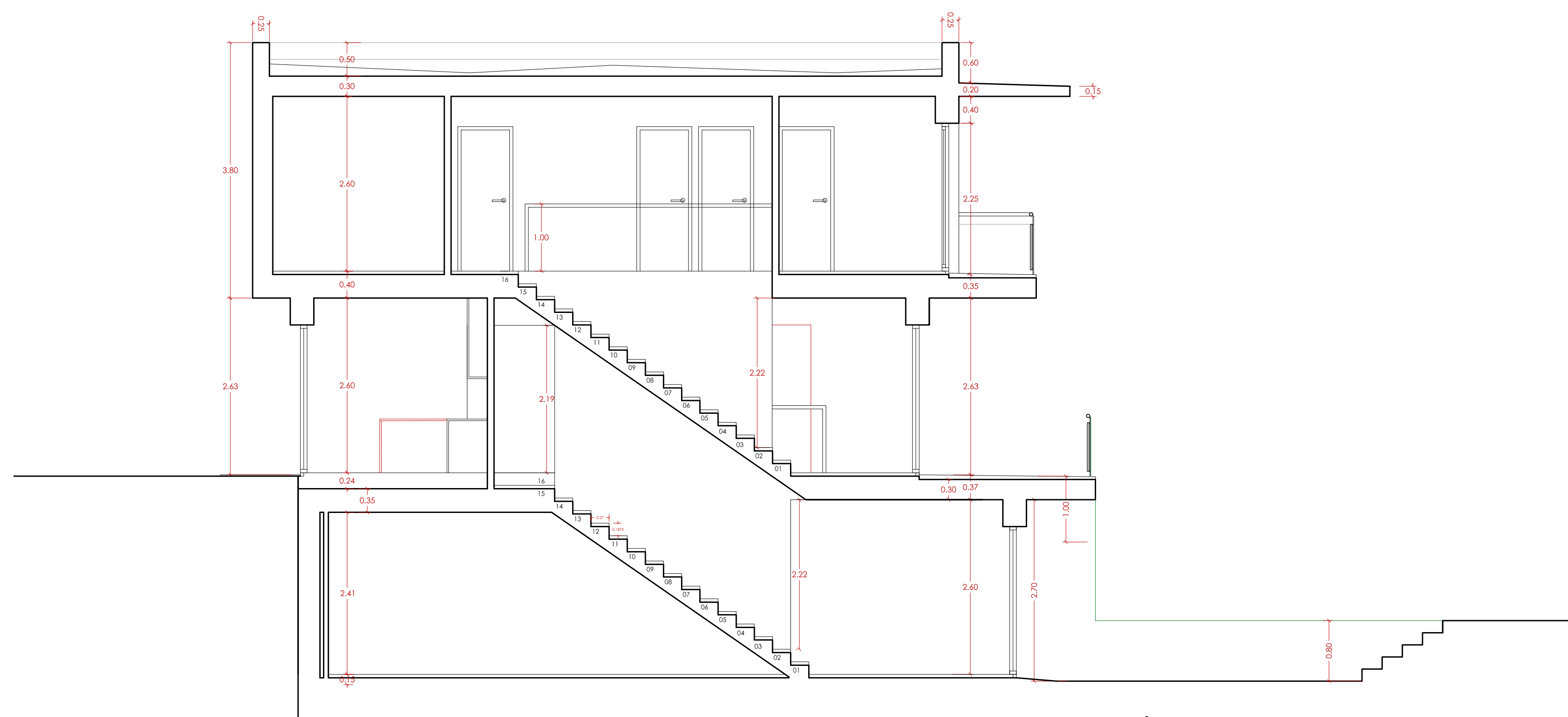
SECCIÓN A-A'
